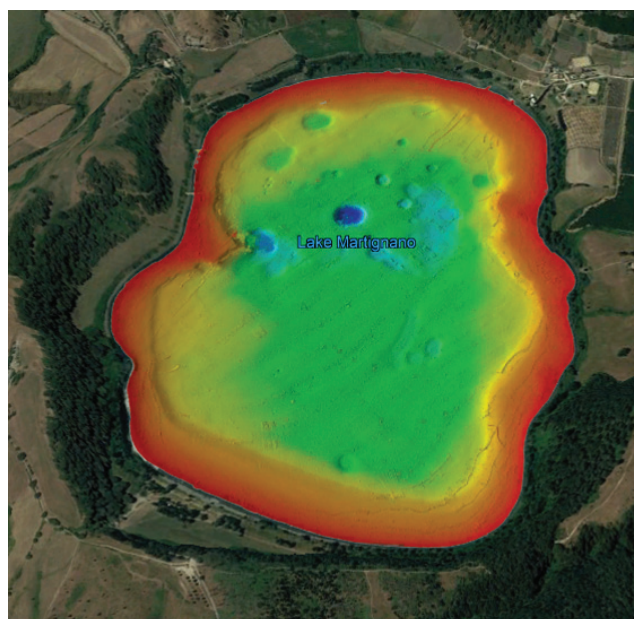
Fig. 5 - Carta batimetrica del Lago di Martignano (rilievi inediti CMRC 2020).
