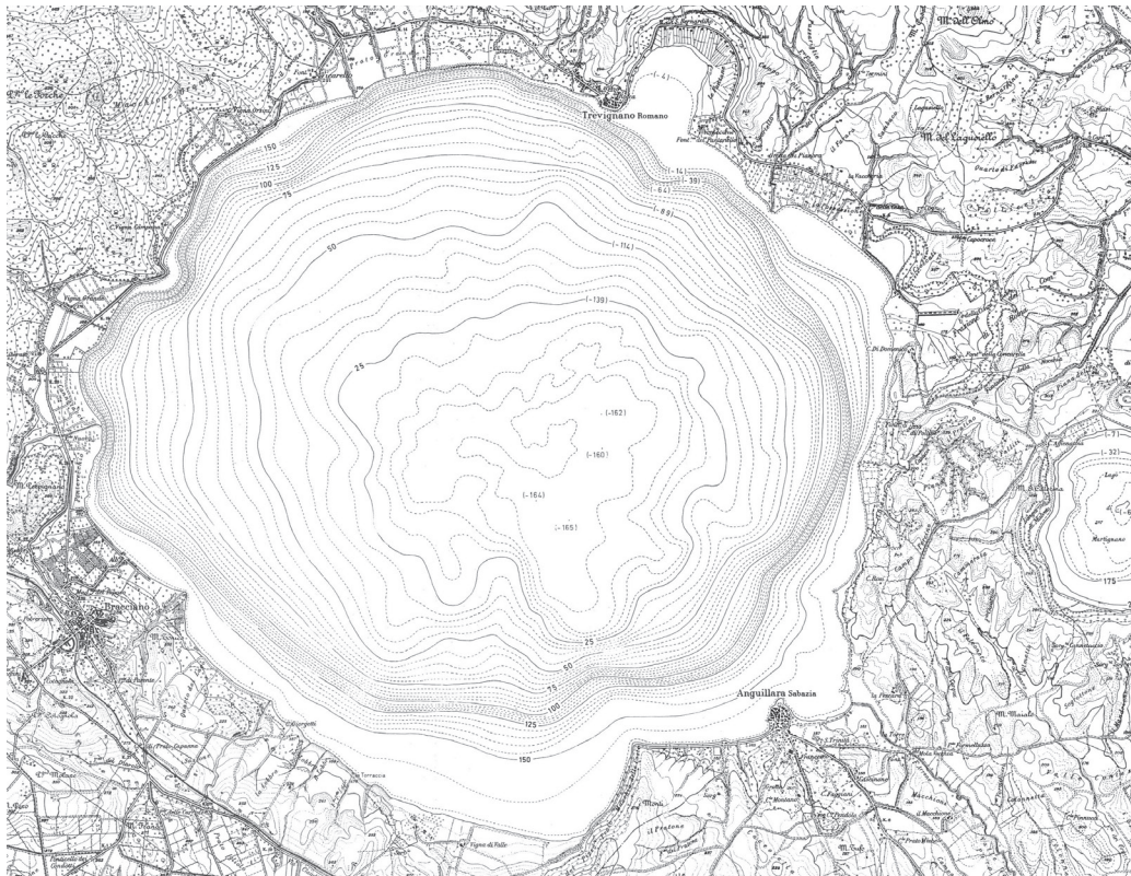
Fig. 2 - Batimetria del Lago di Bracciano (da Barbanti & Carollo 1969).
