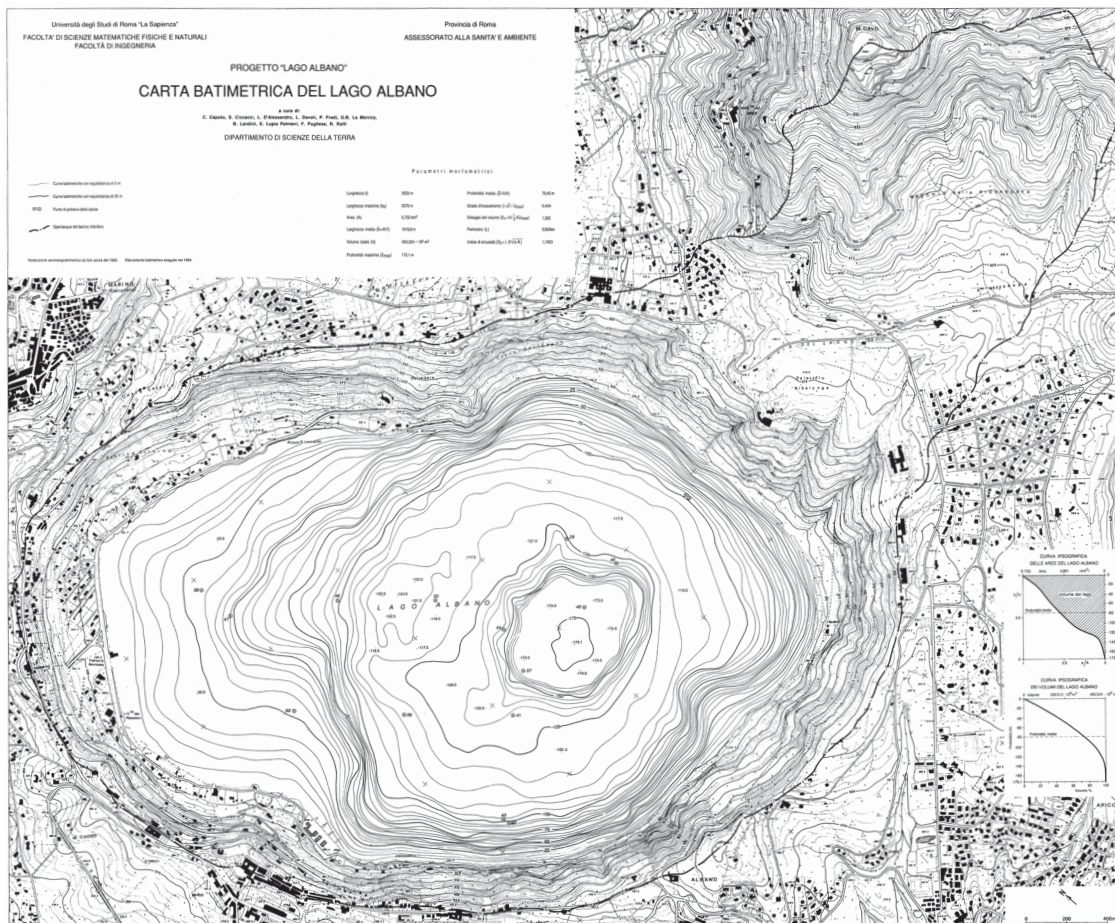
Fig. 3 - Batimetria del Progetto "Lago Albano" (da Caputo et al. 1986).
